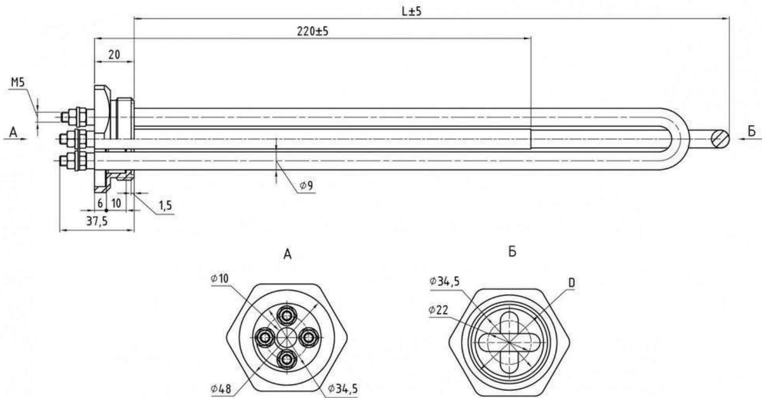
Блок трубчастих електронагрівачів прямий
